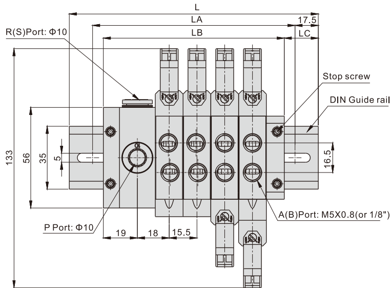
6HV100M2F~10F Guide rail
