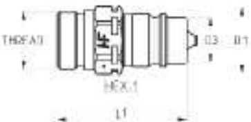
CNVHF
