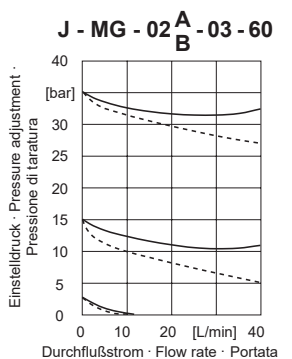
Bild / Fig. 8 — 70 bar - - - 250 bar
