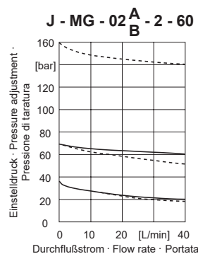
Bild / Fig. 10 — 160 bar - - - 250 bar
