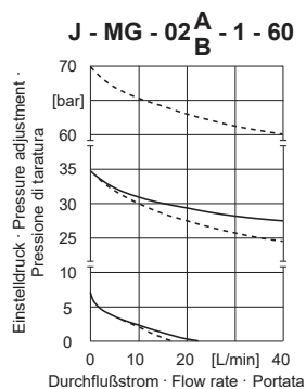
Bild / Fig. 9 — 70 bar - - - 250 bar
