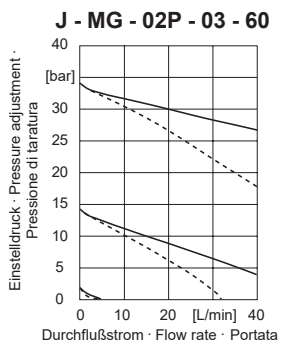
Bild / Fig. 5 — 70 bar - - - 250 bar
