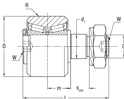
Eccentric PK
