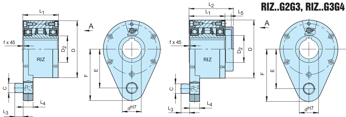
RIZ...G2G3
