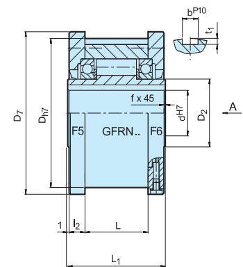
GFRN..F5F6
