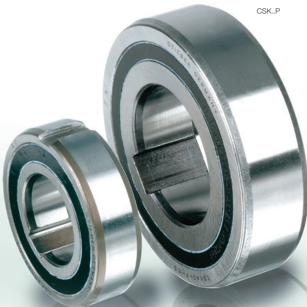
CSK..PP
