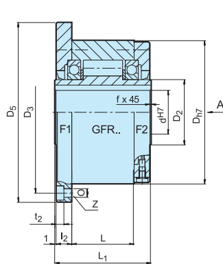
GFR..F1F2
