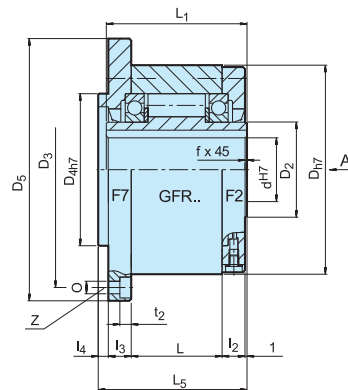
GFR..F2F7
