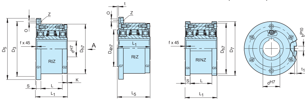
RIZ...G1G2
