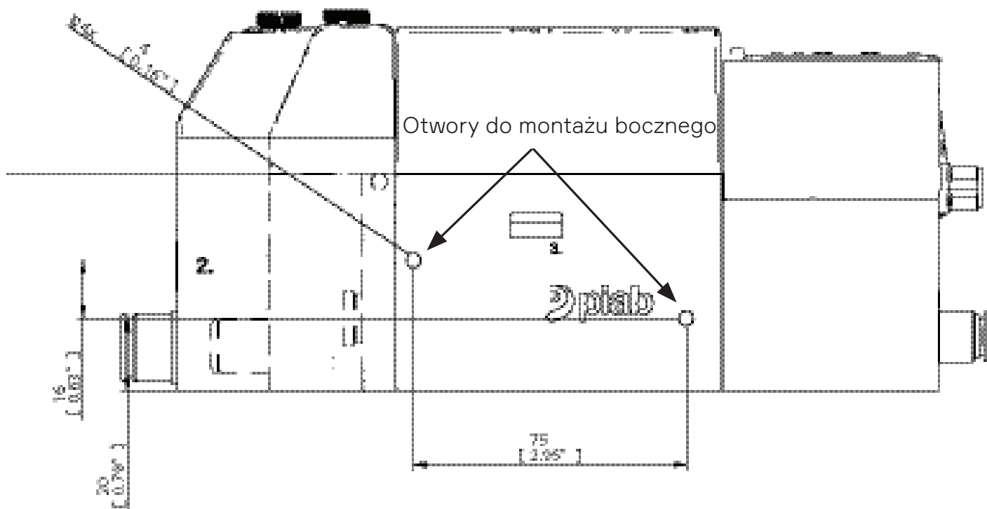
Figure 13 Montaż boczny, 1 kanał.
