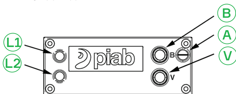
Figure 9 Moduł zaworów.
