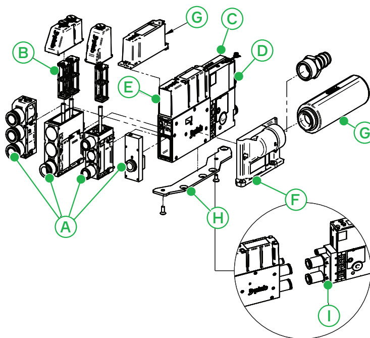
Figure 1 Przegląd, IO-Link, 1 kanał
