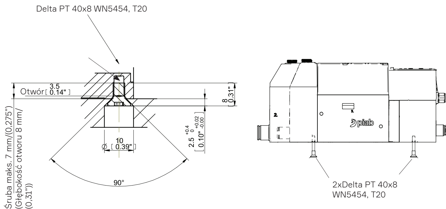
Figure 11 Z filtrem.
