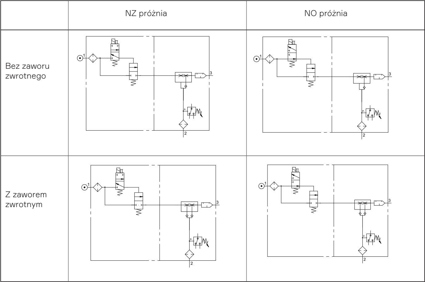
Figure 3 1. Sprężone powietrze, 2. Próżnia, 3. Wylot.
