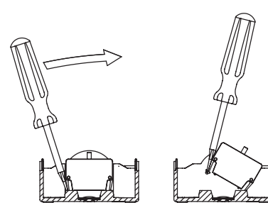
Déclenchage du bloc de contact du fond du boîtier
