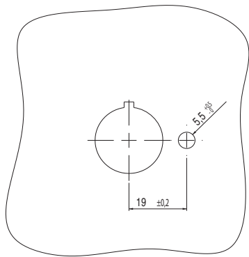
A: Trou pour le passage des câbles
