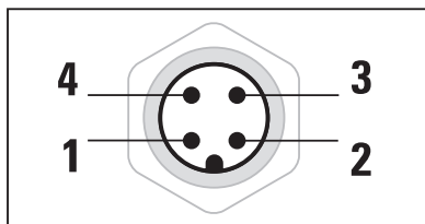
Schemazeichnung M12-Stecker
