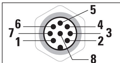
Disegno schematico connettore 12
