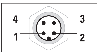
Disegno schematico connettore M12
