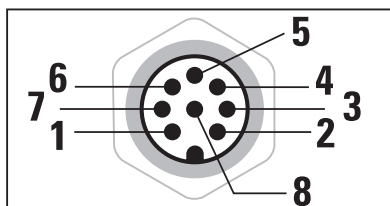
Diagrama del conector M12
