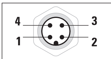
Schéma du connecteur M12
