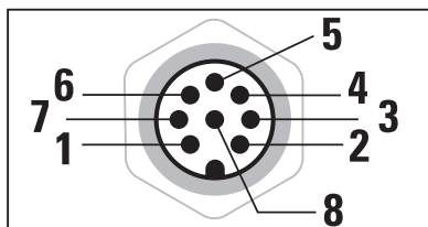
Schemazeichnung M12-Stecker
