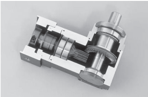
PowerTRUE Gear
