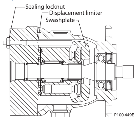
Displacement limiter M35/M44 MV
