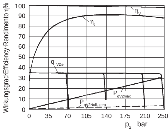
Bild / Fig. 15: Baugröße · Model · Grandezza J-V23 A SA A-RC D
