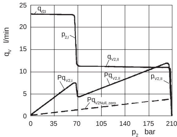
Bild / Fig. 13: Baugröße · Model · Grandezza J-V15 CH
