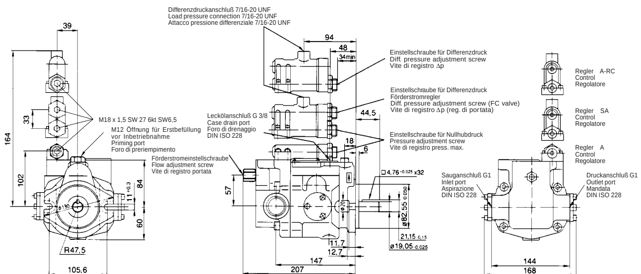
Bild / Fig. 36: Baugröße · Model · Grandezza J-V15 A*RX
