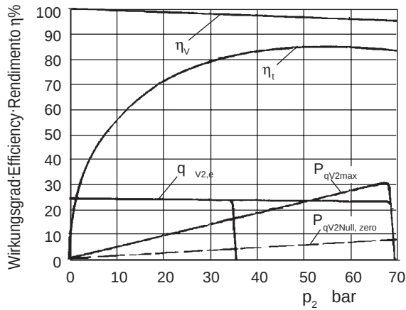
Bild / Fig. 11: Baugröße · Model · Grandezza J-V8 A
