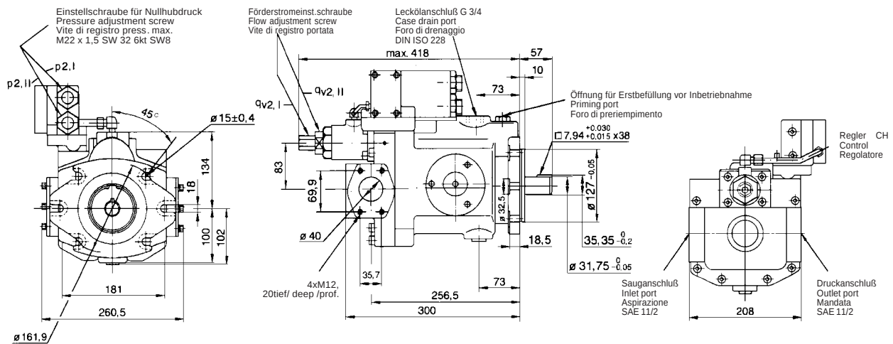
Bild / Fig. 53: Baugröße · Model · Grandezza J-V70C**RH
