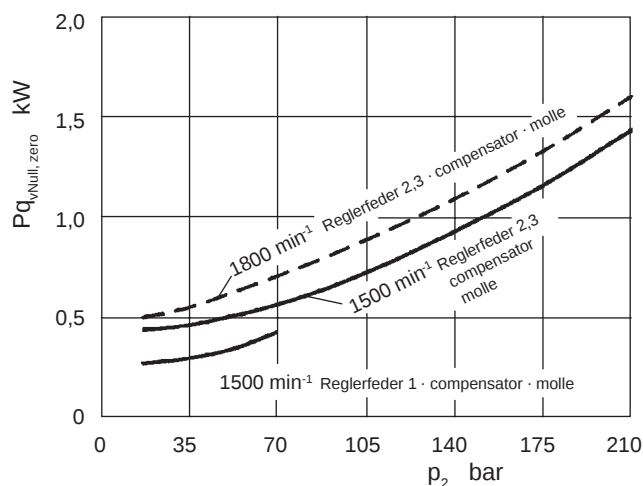
Bild / Fig. 30: Baugröße · Model · Grandezza J-V15
