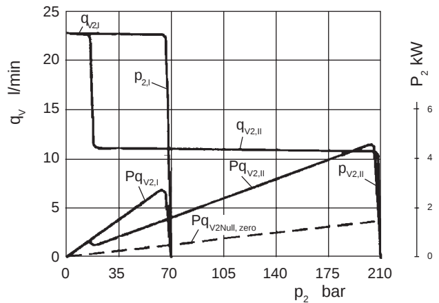
Bild / Fig. 14: Baugröße · Model · Grandezza J-V15CJ
