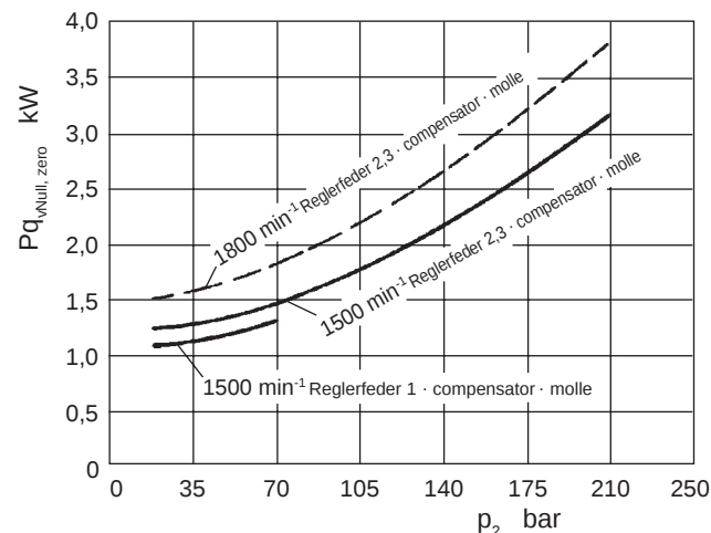
Bild / Fig. 34: Baugröße · Model · Grandezza J-V70
