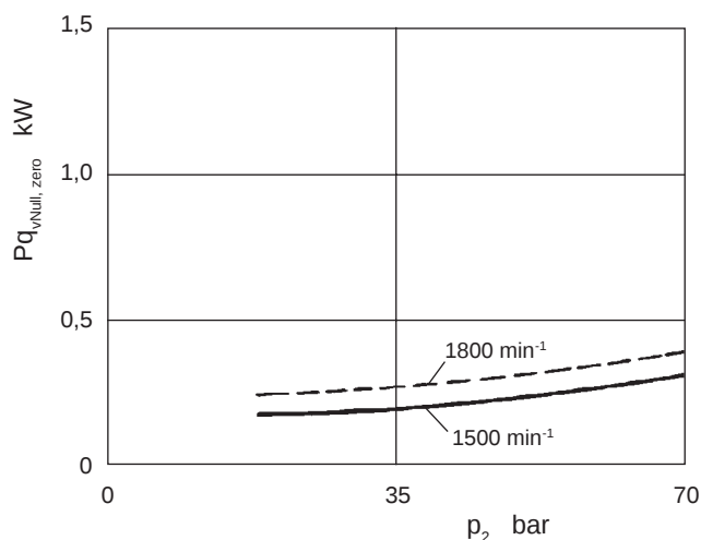
Bild / Fig. 29: Baugröße · Model · Grandezza J-V8
