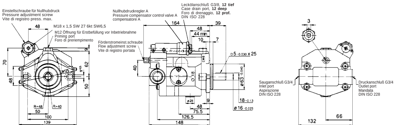
Bild / Fig. 35: Baugröße · Model · Grandezza J-V8A*RX
