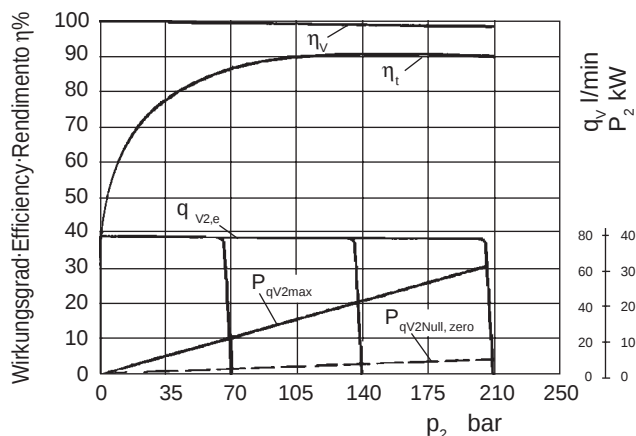
Bild / Fig. 21: Baugröße · Model · Grandezza J-V50 A SA A-RC
