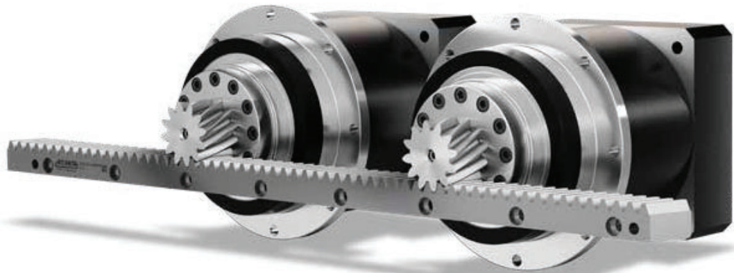
Mehrfachzahneingriff zur elektronischen Verspannung Multiple pinion contact for electronic preload
