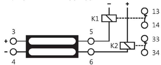
BILD 2. NICHT AKTIVIERTES SENSORELEMENT
