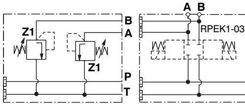
Gegenseitig unabhängige Druckabsicherung im Kanal A, B
