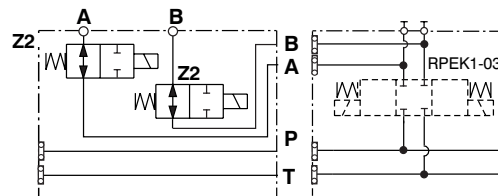
Block mit 2/2-Schieber-Wegeventilen
