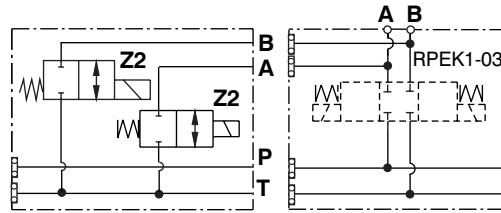
Entlastungsventile in Kanälen A, B
