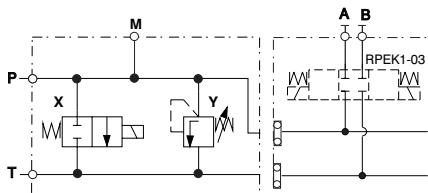
Versorgungsblock mit Druckbegrenzungsventil und 2/2-Wegeventil für drucklosen Umlauf
