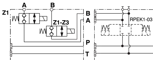
Block mit Sitzventilen
