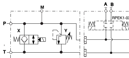
Versorgungsblock mit Druckbegrenzungsventil und 2/2-Wegesitzventil für drucklosen Umlauf
