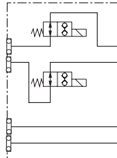
Block mit Sitzventilen
