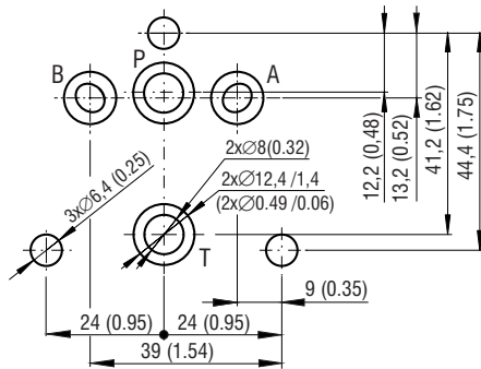
Anschlussbild für horizontale Verkettung
