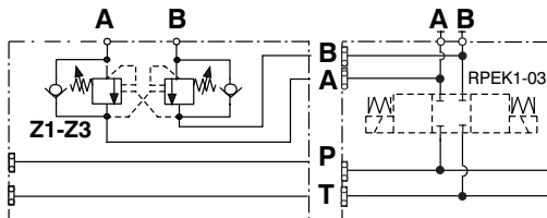
Block mit Senkbremsventilen
