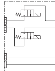
Block mit Schieber-Wegeventilen
