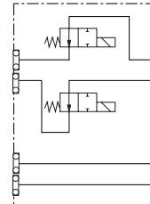
Block mit Schieber-Wegeventilen
