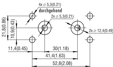
Anschlussbild für vertikale Verkettung
