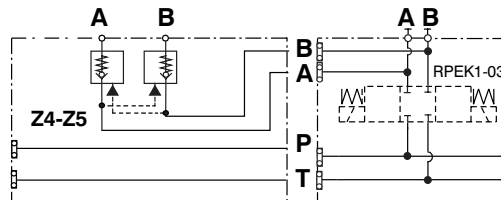
Block mit entsperrbaren Rückschlagventilen
