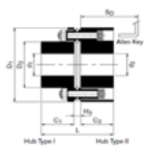
RLDS BWB: Ara Parçasız Tek Mafsallı
