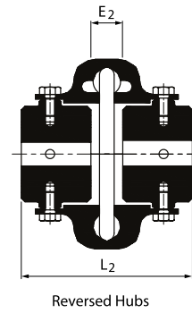
RLU RWR Göbek Ters Çevrilmiş Tip
