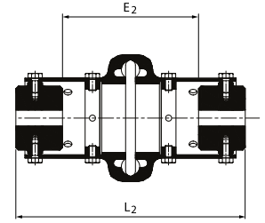
RLU RSR Göbek Ters Çevrilmiş Tip
