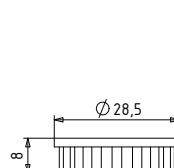
Rändelmutter Knurled nut
