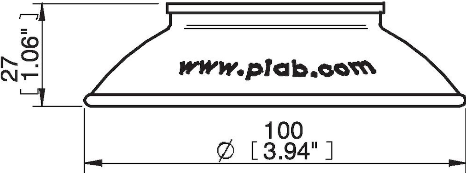
Rysunki wymiarowe
