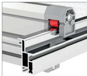
vedení příčnicku
