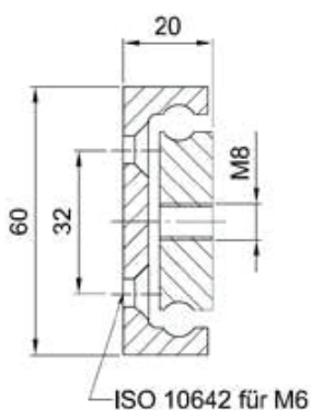
NTA60-20
