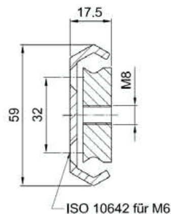
NTA59-17.5T
