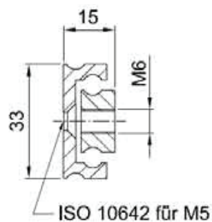
NTA33-15
