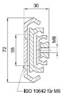
NTU72-30T
