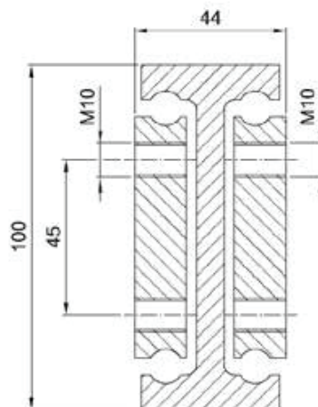
NTS100-44
