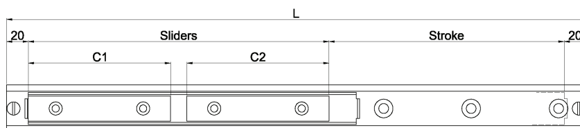
LSS43-L Gesamtlänge – Hub – 2 x Länge der Gleitschiene
