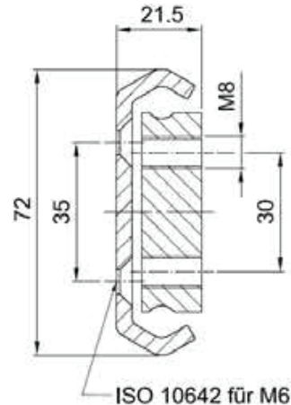
NTA72-21.5T
