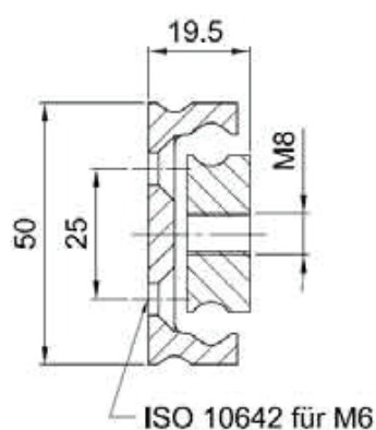
NTA50-19.5
