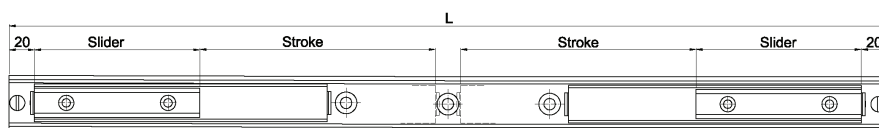
LSS43-L Gesamtlänge-Doppelhub
