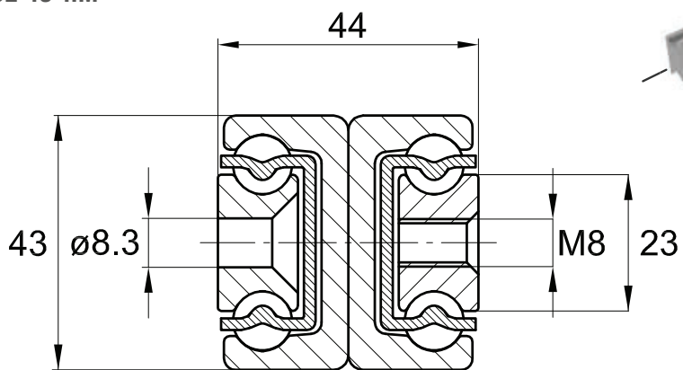
LSE 43-..M
