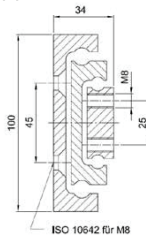
NTV100-34
