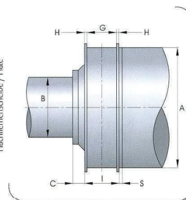
Piana / Flat Flachriemenscheibe / Plate
