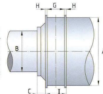
Piana / Flat Flachriemenscheibe / Plate
