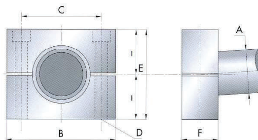
Supporto fisso a base tipo FB Fixed base type support: FB Feste Fußlagerung Typ FB Support fixe à socle type FB
