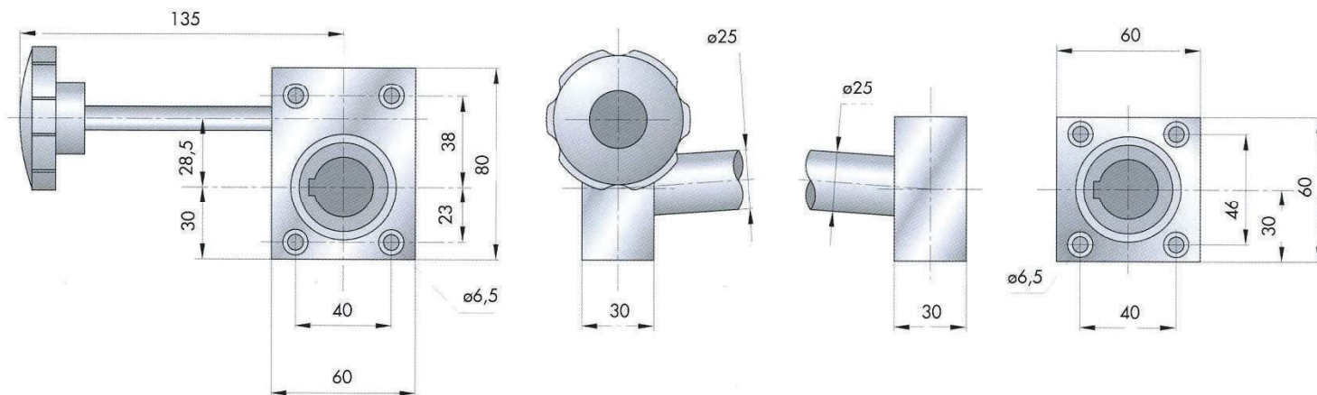
Supporto rotante serie RM / Rotating support RM Rotierende Lagerung Typ RM / Support tournant série RM
