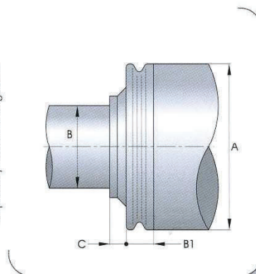
Testata a sgocciolo / Drip head Tropfenle / Extrémité à égouttoir
