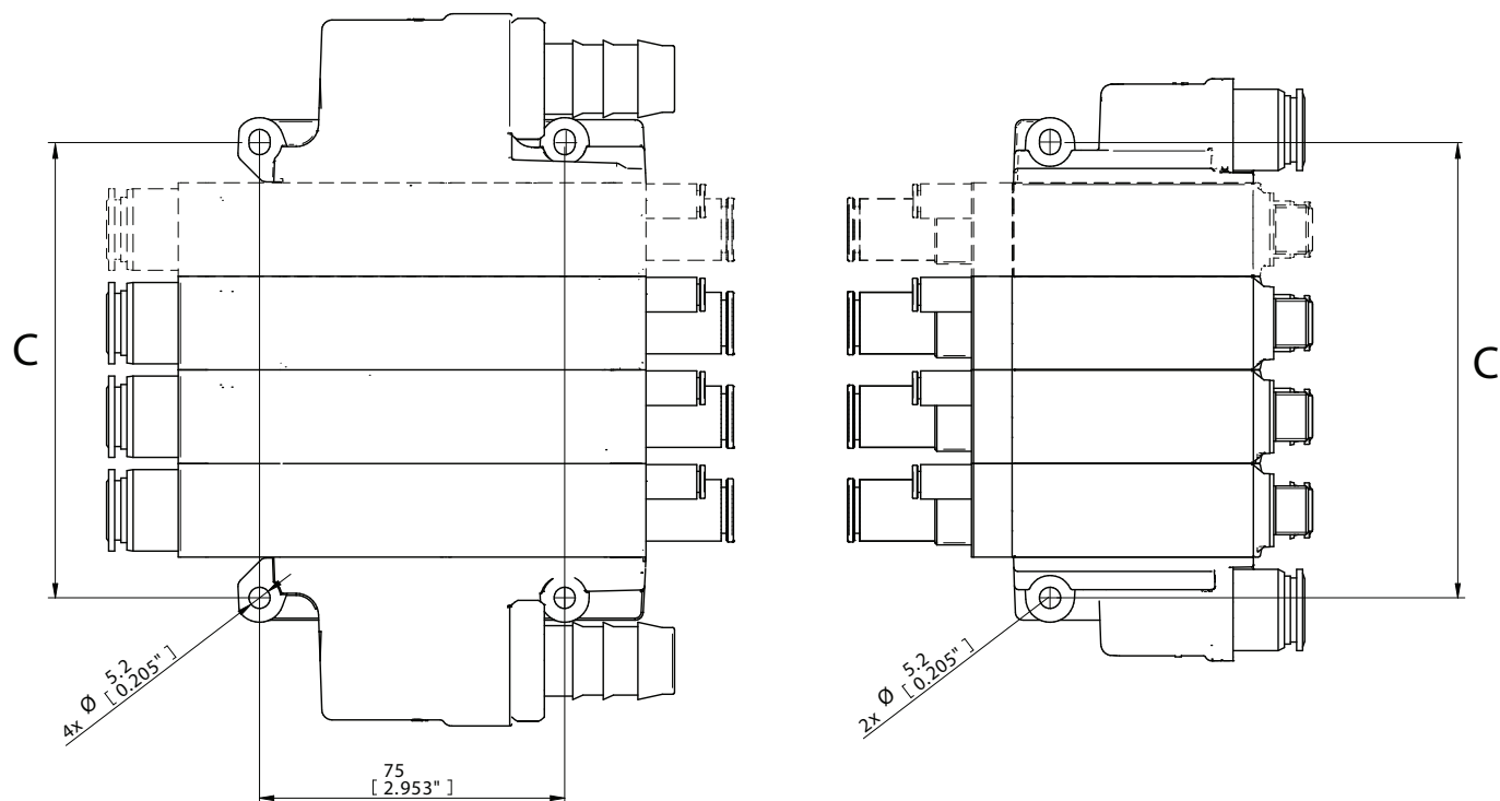
Figure 11 Podział, mocowanie kolektora.
