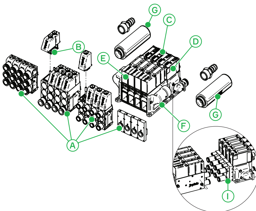
Figure 1 Przegląd, IO-Link, 3–4 kanały
