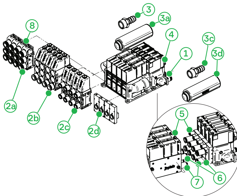
Figure 2 Przyłącza, 3–4 kanały
