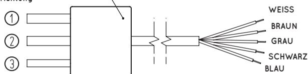
Verteiler mit integrierter Energiesparvorrichtung
