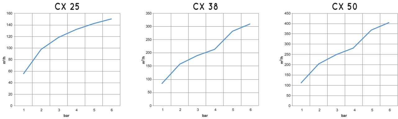
Blasluftmenge (m 3 /h) bei unterschiedlichen Versorgungsdrücken (bar)
