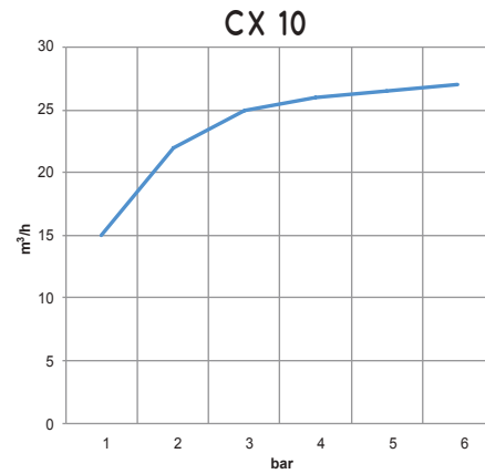
Blasluftmenge ( \text{m}^3/\text{h} ) bei unterschiedlichen Versorgungsdrücken (bar)
