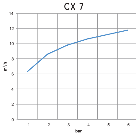
Blasluftmenge ( \text{m}^3/\text{h} ) bei unterschiedlichen Versorgungsdrücken (bar)
