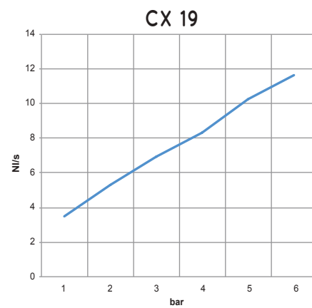
Luftverbrauch ( \text{NI/s} ) bei unterschiedlichen Versorgungsdrücken (bar)
