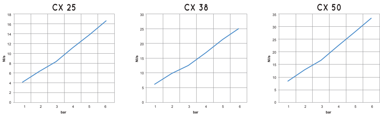
Luftverbrauch (Nl/s) bei unterschiedlichen Versorgungsdrücken (bar)
