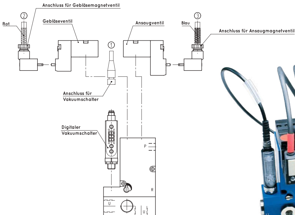
Verteiler mit integrierter Energiesparvorrichtung
