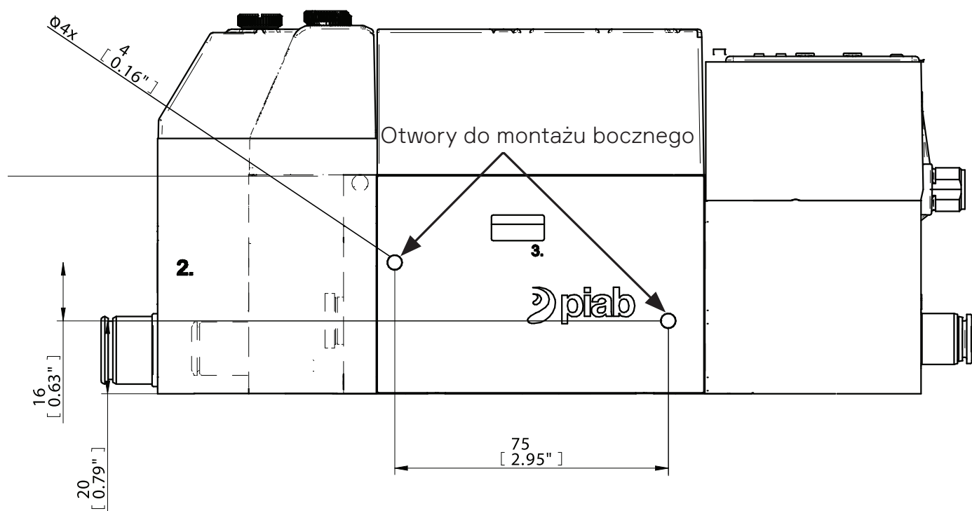
Figure 13 Montaż boczny, 1 kanał.
