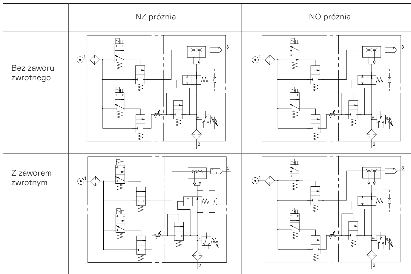
Figure 4 1. Sprężone powietrze, 2. Próżnia, 3. Wylot.
