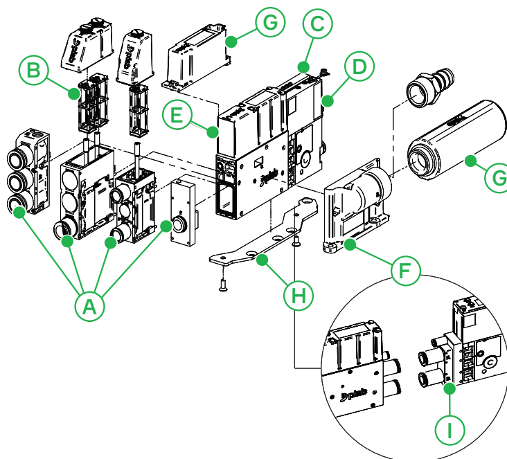
Figure 1 Przegląd, wersja 1-kanałowa.
