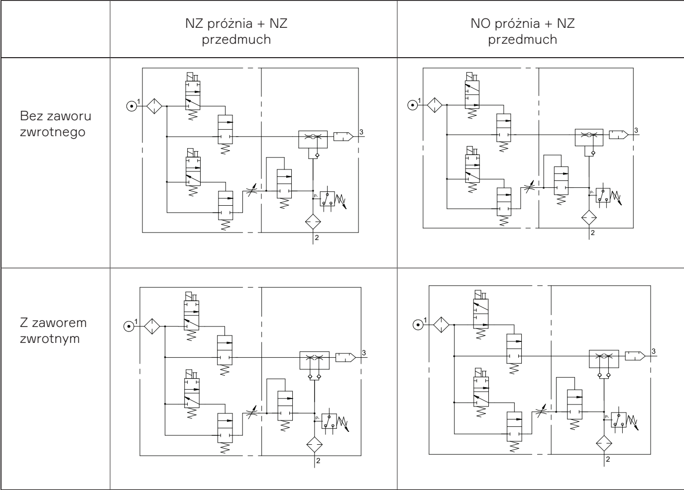
Figure 3 1. Sprężone powietrze, 2. Próżnia, 3. Wylot.
