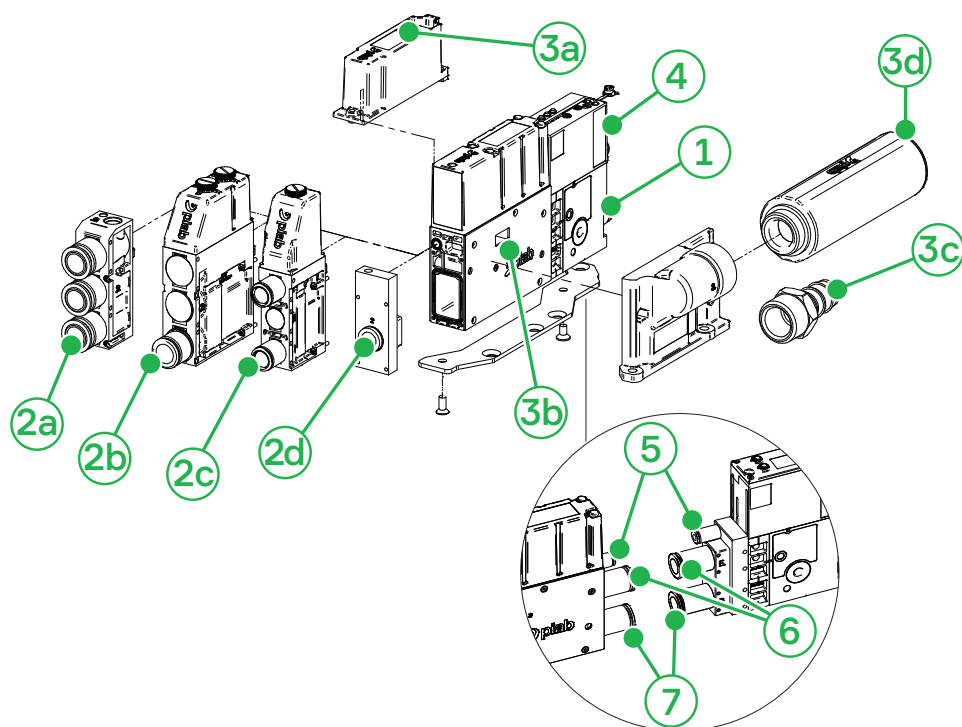
Figure 2 Połączenia, 1 kanał.
