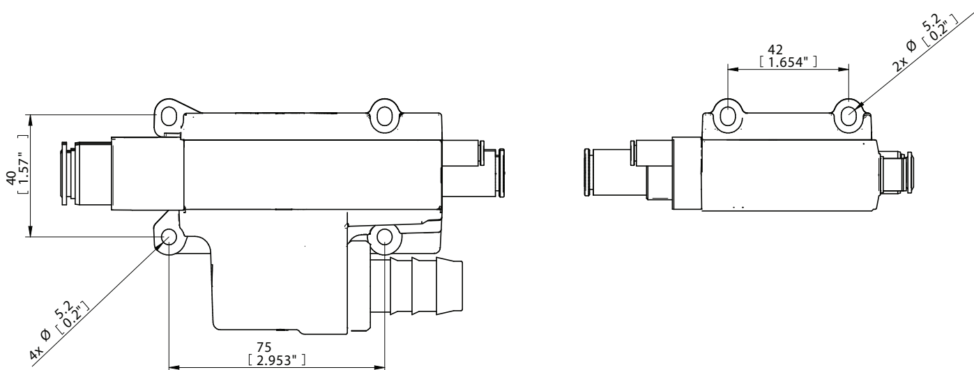
Figure 16 Podział, mocowanie kolektora
