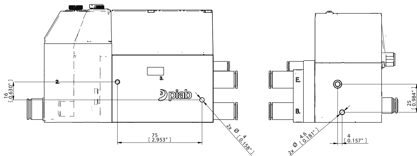
Figure 14 Interfejs do montażu bocznego, podział
