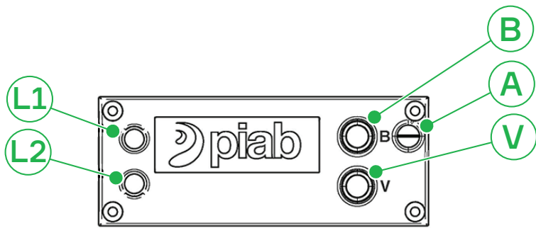
Figure 9 Moduł zaworów.
