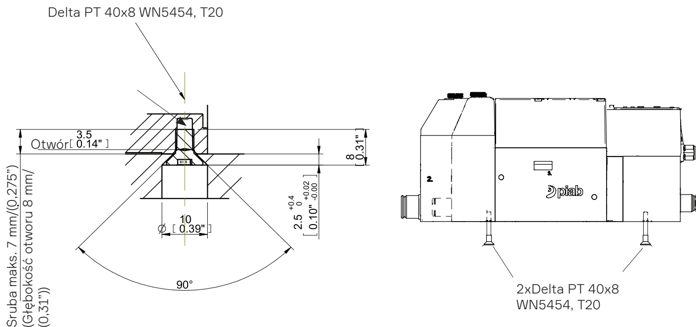
Figure 11 Z filtrem.
