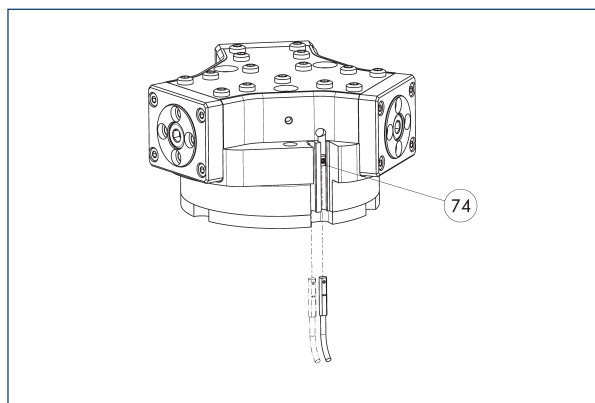
⑦④ Koncová zarážka pro snímač
