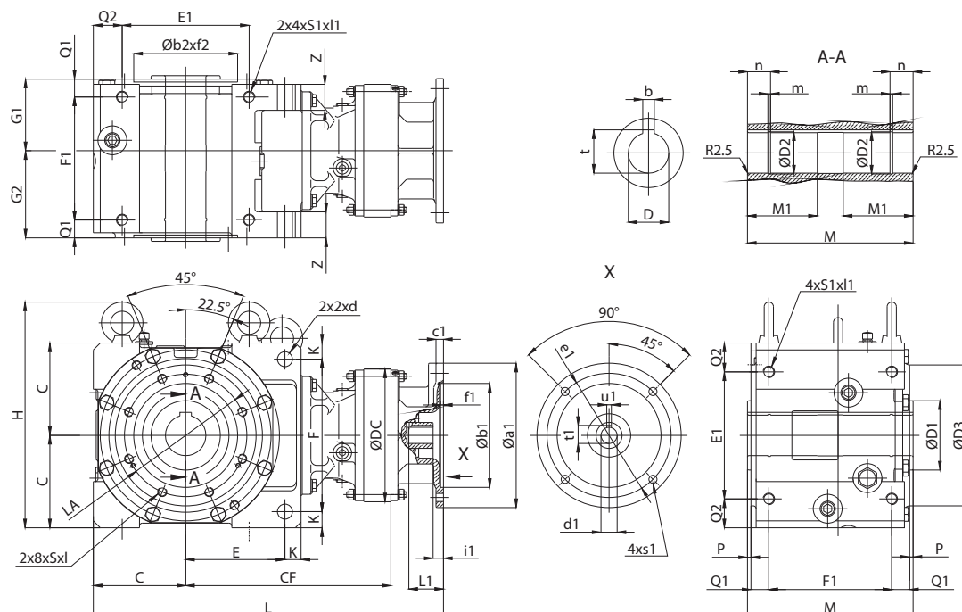
Example/Beispiel: LHYX-3B125EY1-178/90/A200
