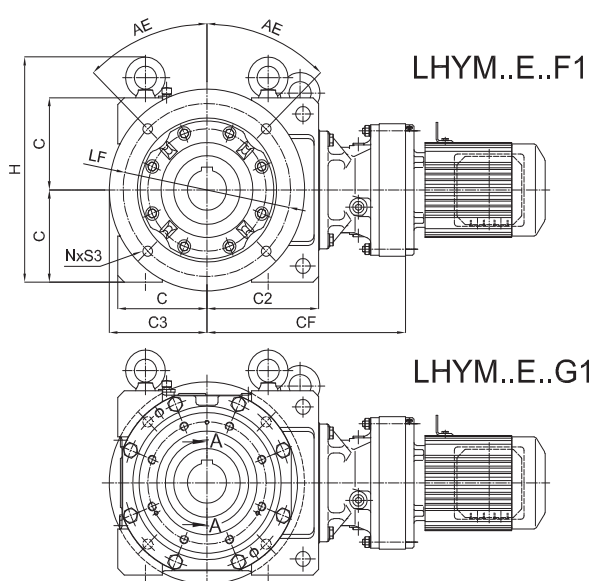
Example/Beispiel: LHYM2-3B145EF1-249/V90L/4
