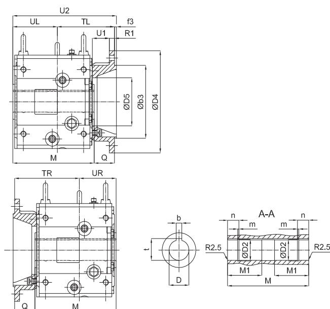
Example/Beispiel: LHYM2-3B145EF1-249/V90L/4
