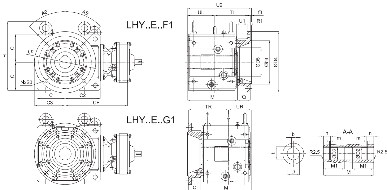
Example/Beispiel: LHY-3B125EF1-179
