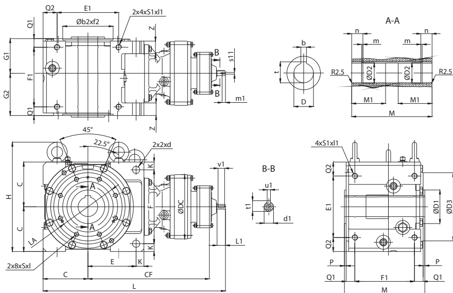
Example/Beispiel: LHY-3D16DBEY1-578
