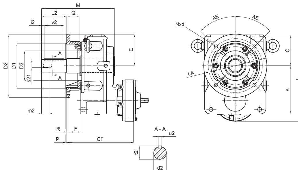
Example/Beispiel: EHF-A6105EP3-21
