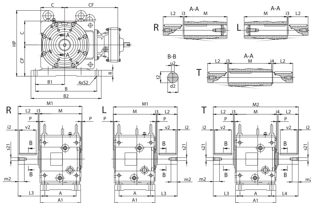
Example/Beispiel: LHH-3B125LES1-179
