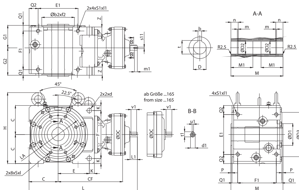
Example/Beispiel: LHY-3B125EY1-179
