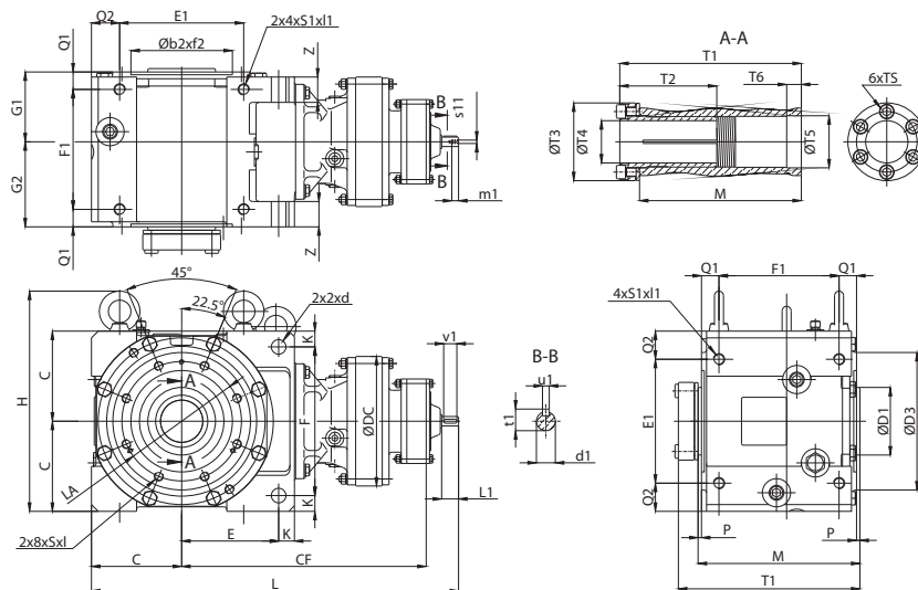
Example/Beispiel: LHY-3D16DBGY1-578
