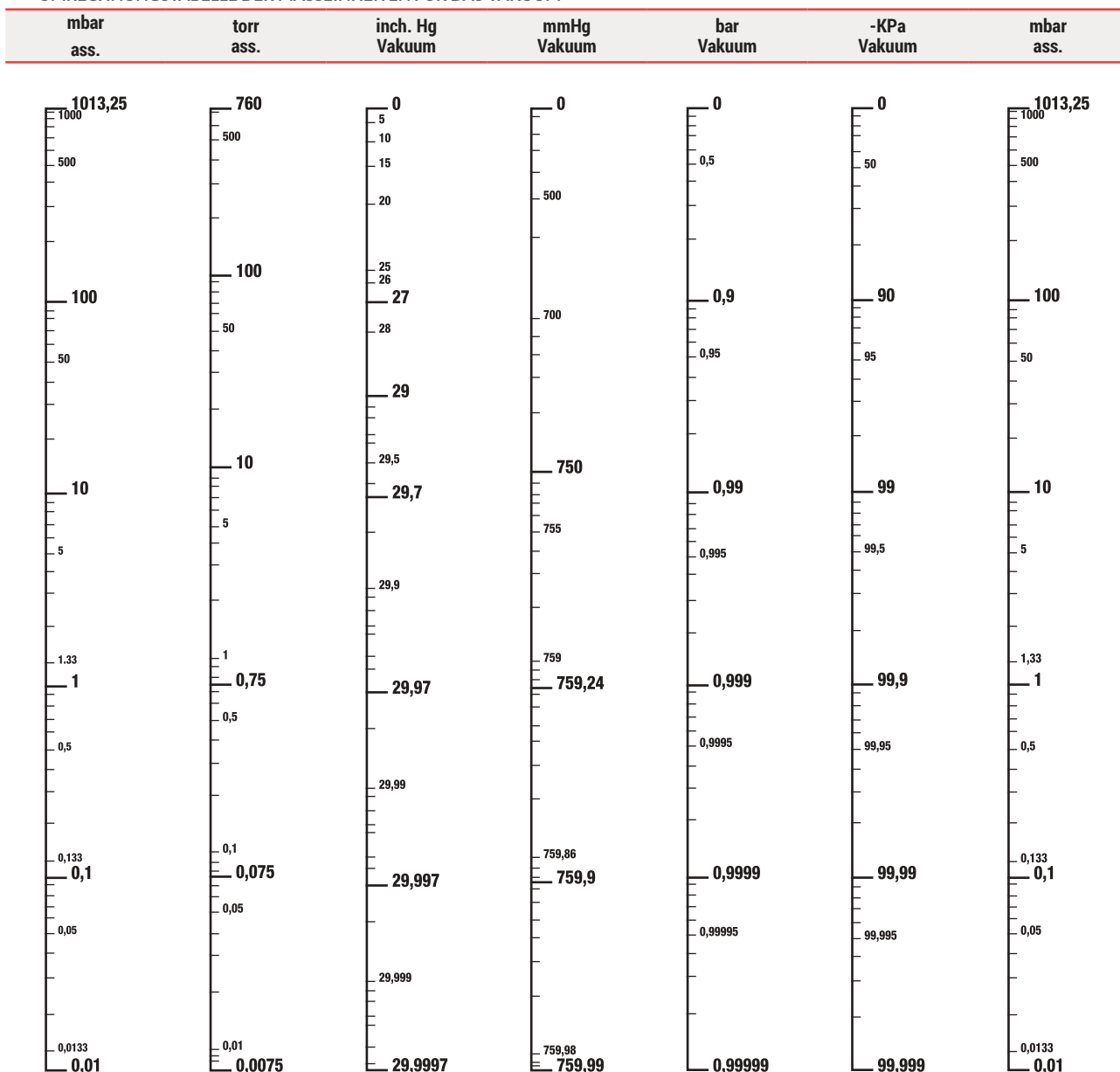
UMRECHNUNGSTABELLE DER MASSEINHEITEN FÜR DAS VAKUUM
