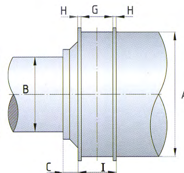
Piana / Flat Flachriemenscheibe / Plate
