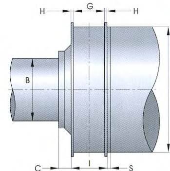
Piana / Flat Flachriemenscheibe / Plate
