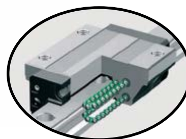
Führungswagen mit Kugellkette
