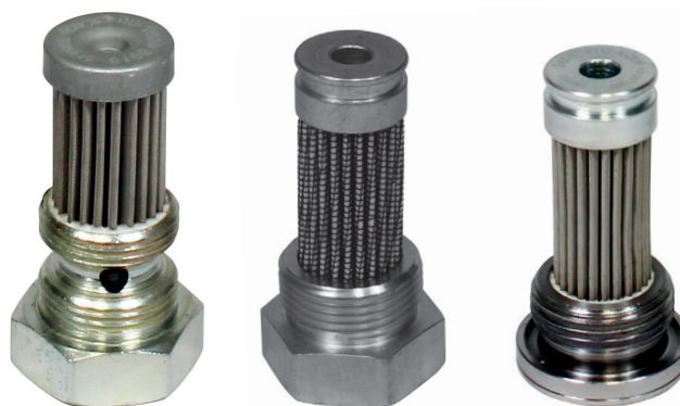
Hochdruck-Filterelement mit integriertem Gewinde
