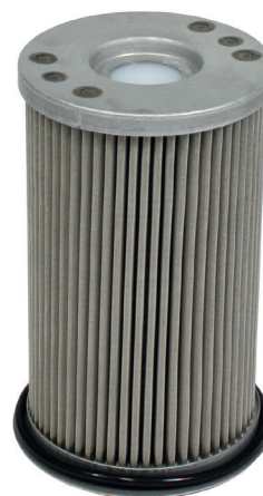
Filterelement mit Bypass und Sonderdichtung
