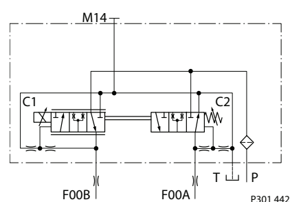
FDC schematic
