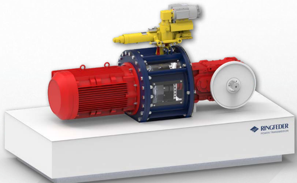
System mit manueller Handspanneinrichtung TZC System with manual clamping device TZC
