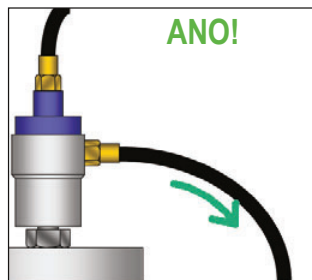
Odtoková hadice má vždy sklon směrem dolů
