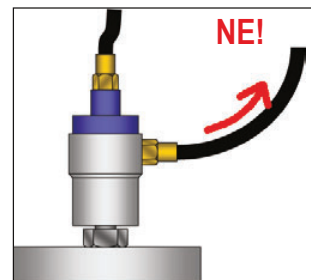
Odtoková hadice směřuje z přívodu nahoru
