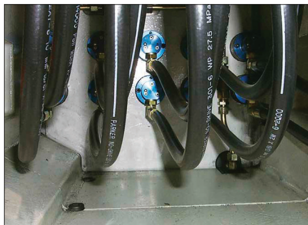
Bezložiskové přívody Deublin 1117 na automobilovém přenosovém potrubí.
