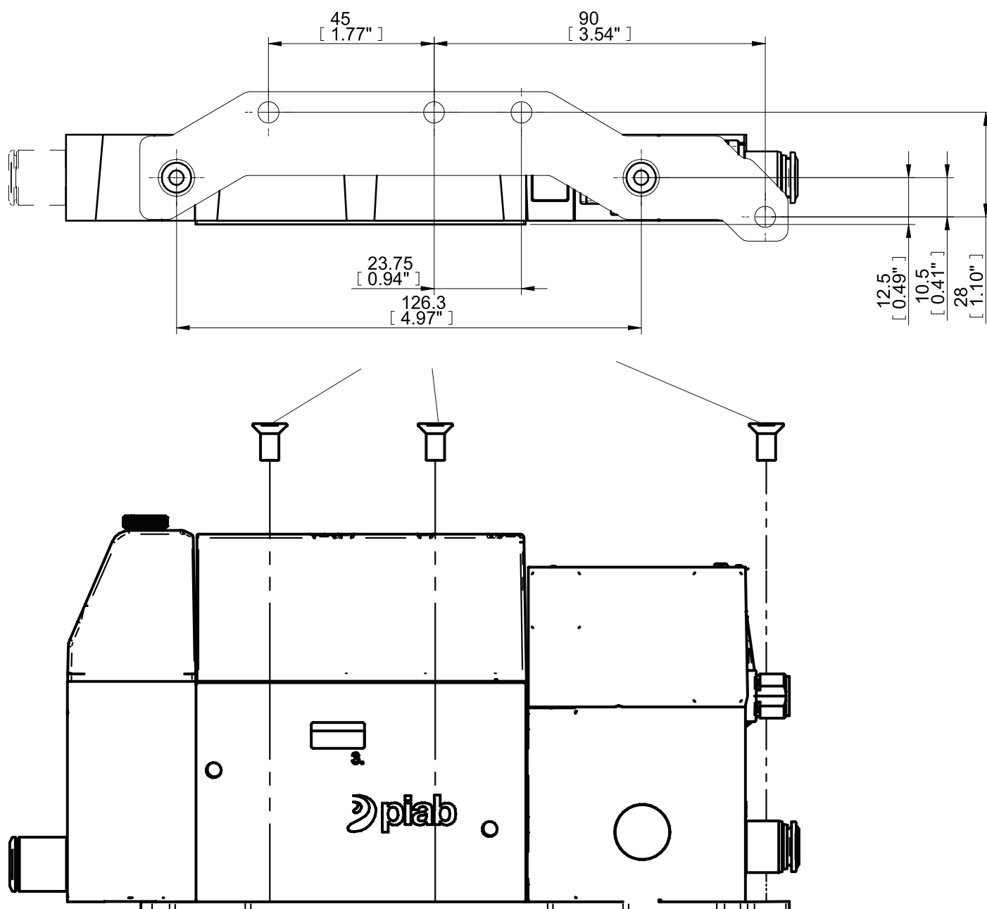
Figure 9 2 kanały.
