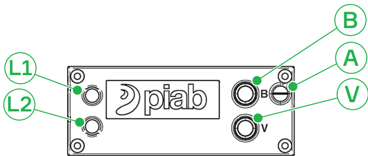
Figure 8 Moduł zaworów.
