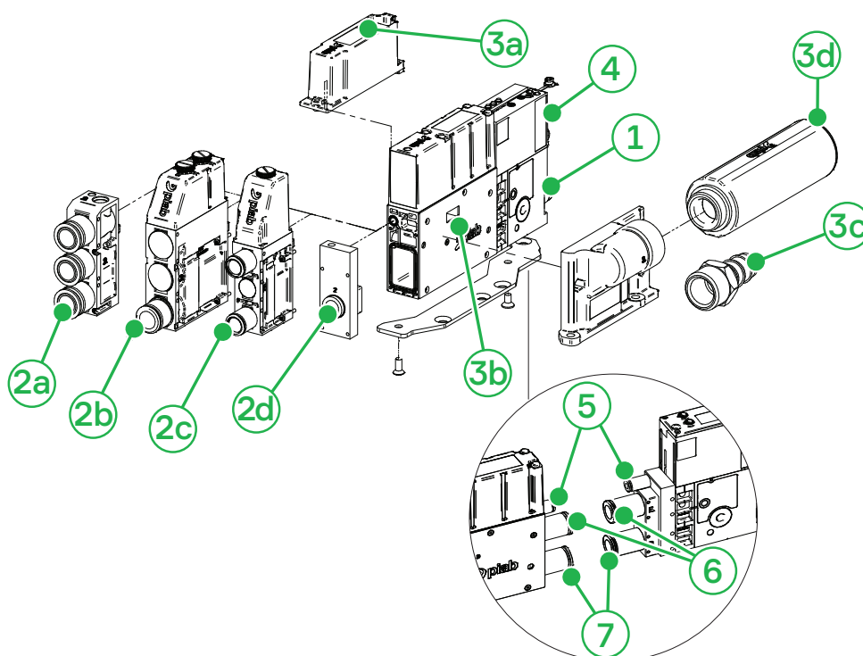
Figure 1 Połączenia, 2 kanały.
