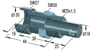
BV25 Bolzenvorlagerung
