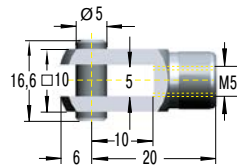
D5-VA Gabelkopf
