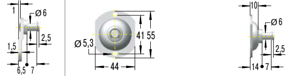
PA5-V4A Rundbeslag
