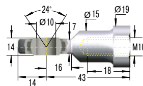
E10-VA Gelenkkopf
