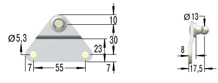
OG8-V4A Seitenbeschlag
