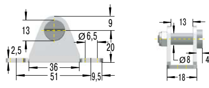
MA10-V4A Lagerschuh
