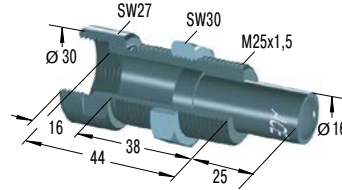
BV25SC Bolzenvorlagerung
