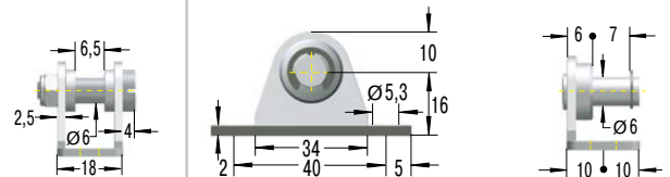
NA5-V4A Winkelbeslag
