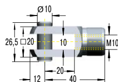
D10-VA Gabelkopf
