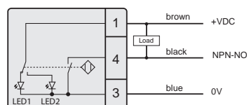
Anschlussbelegung F (NPN) Connection diagram F (NPN)
