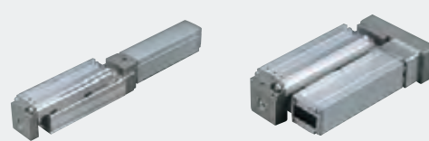
Gerade Ausführung Seitmotor-Ausführung
